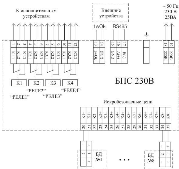
Рисунок 6.12 Монтажная схема БПС 230В.
