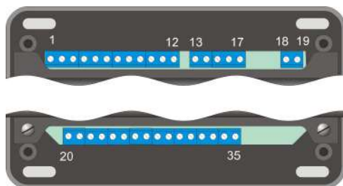
Рисунок 6.11 Клеммы БПС 24В.
