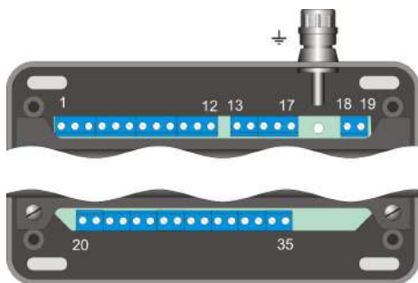
Рисунок 6.10 Клеммы БПС 230В.
