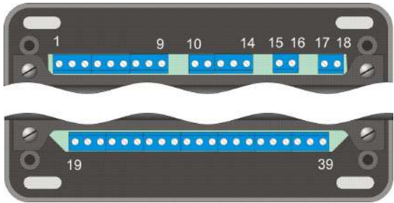
Рисунок 6.14 Клеммы БРР
